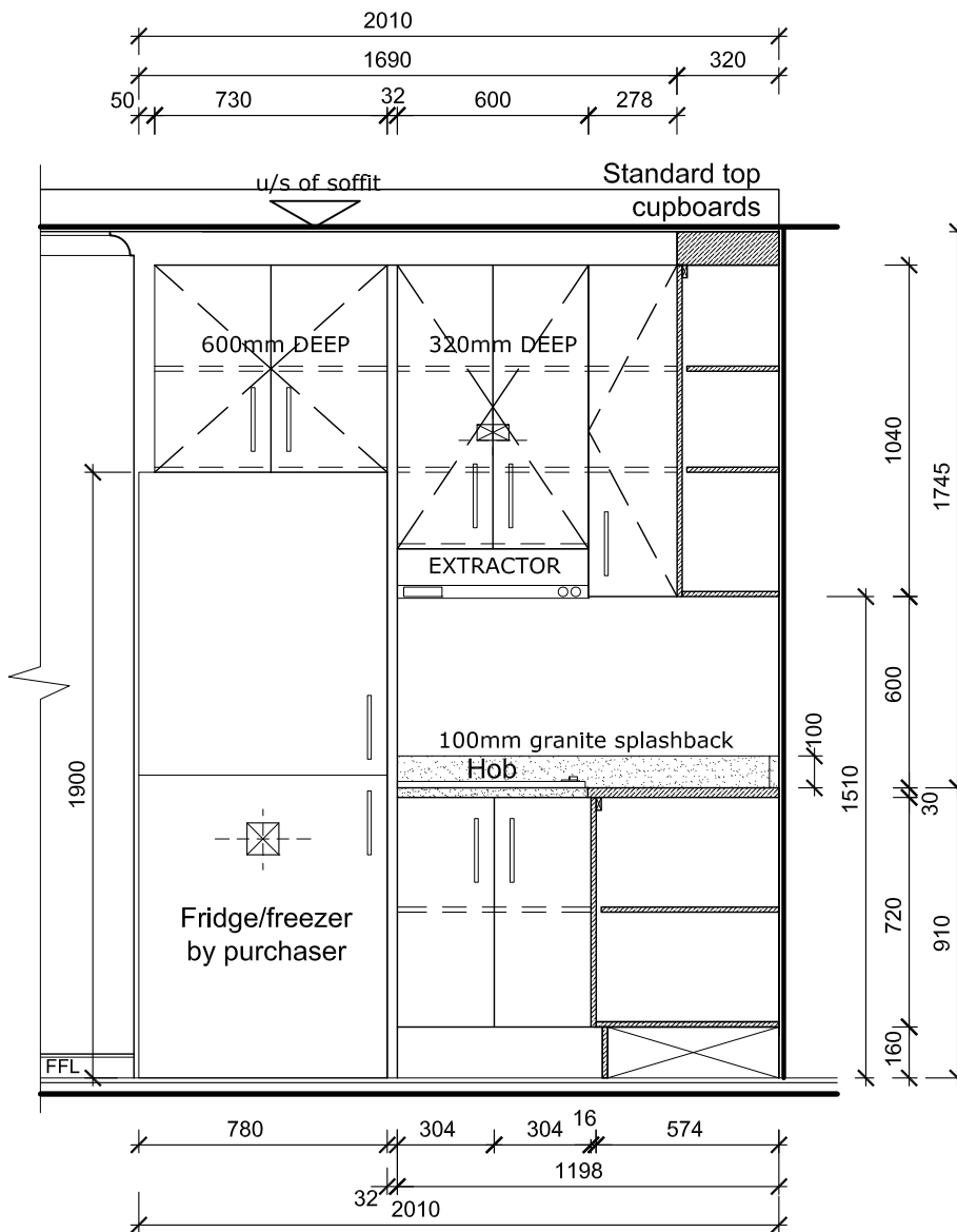
ELEVATION C-C
